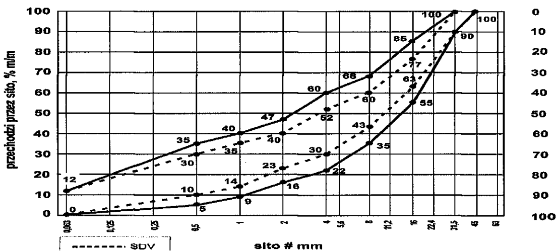
Rys. 1. Uziarnienie mieszanki niezwiązanej 0/31,5 do podbudowy-pomocniczej
