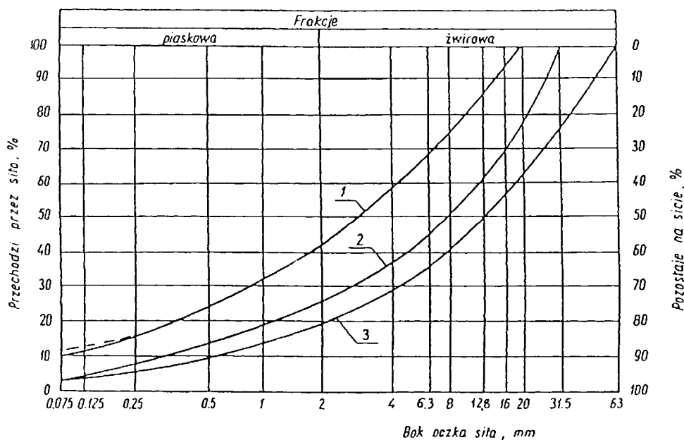
Rysunek 1. Pole dobrego uziarnienia kruszywa przeznaczonych na podbudowy wykonywane metodą stabilizacji
