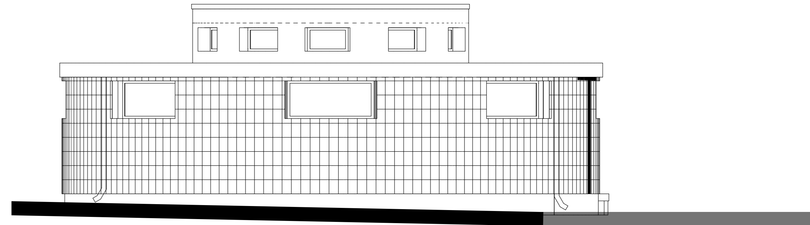
ELEWACJA C-C 1 : 50
