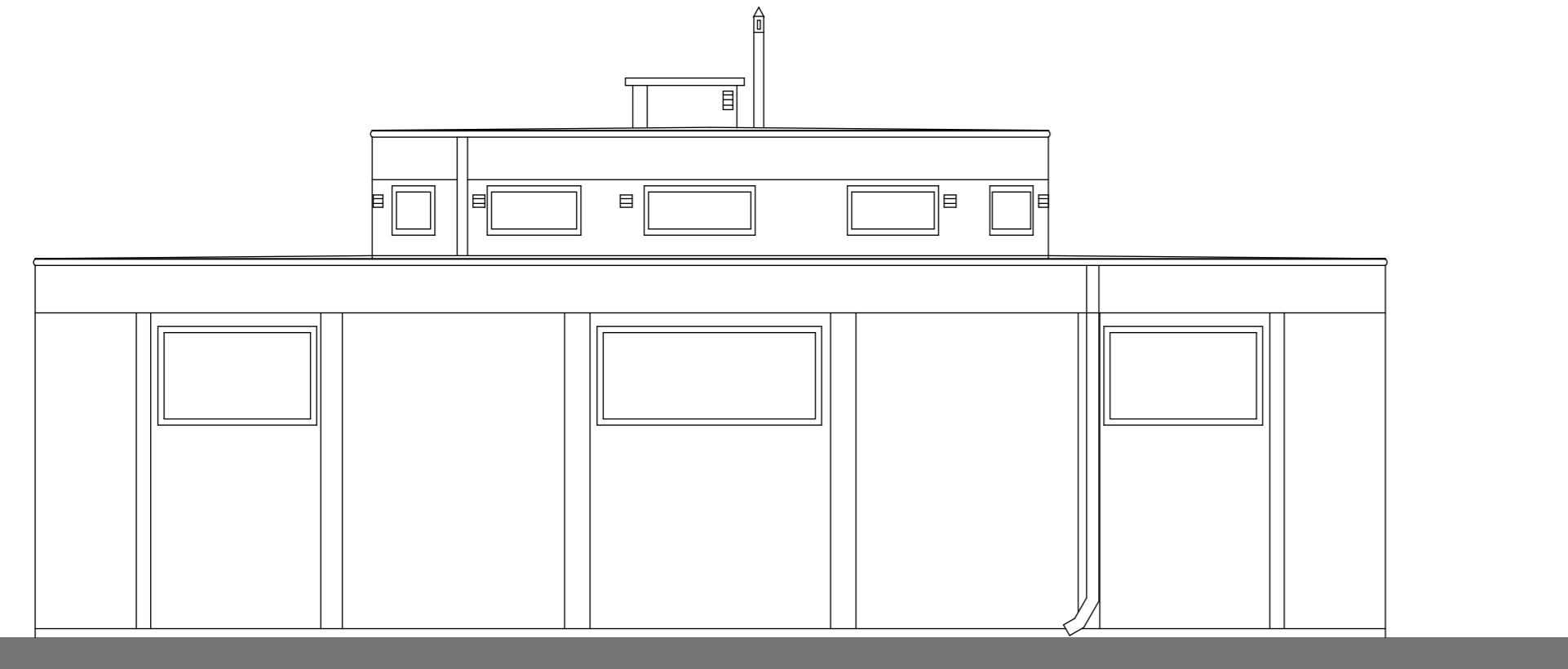
ELEWACJA A-A 1 : 50
